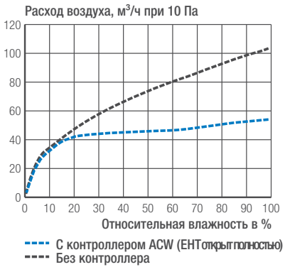
Аэродинамические характеристики
