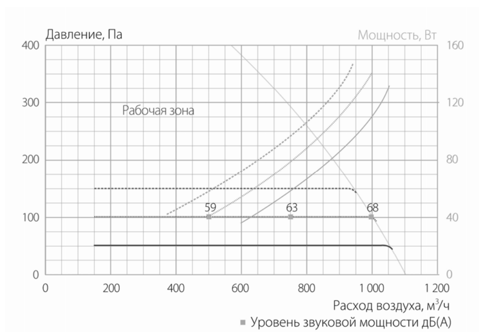
Вентилятор VCZ1085RU
