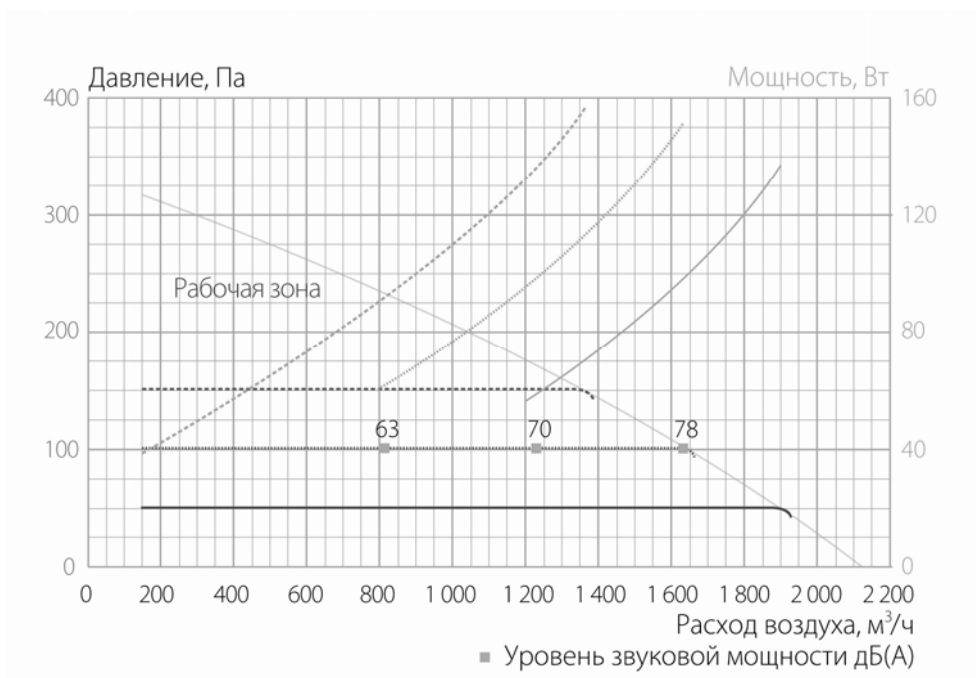
Вентилятор VCZ1086RU
