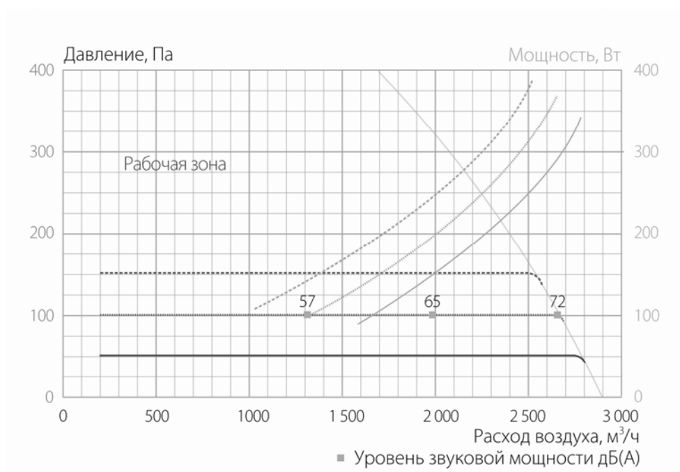
Вентилятор VCZ1087RU
