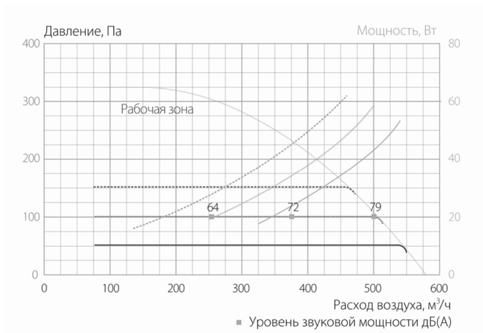
Вентилятор VCZ1084RU
