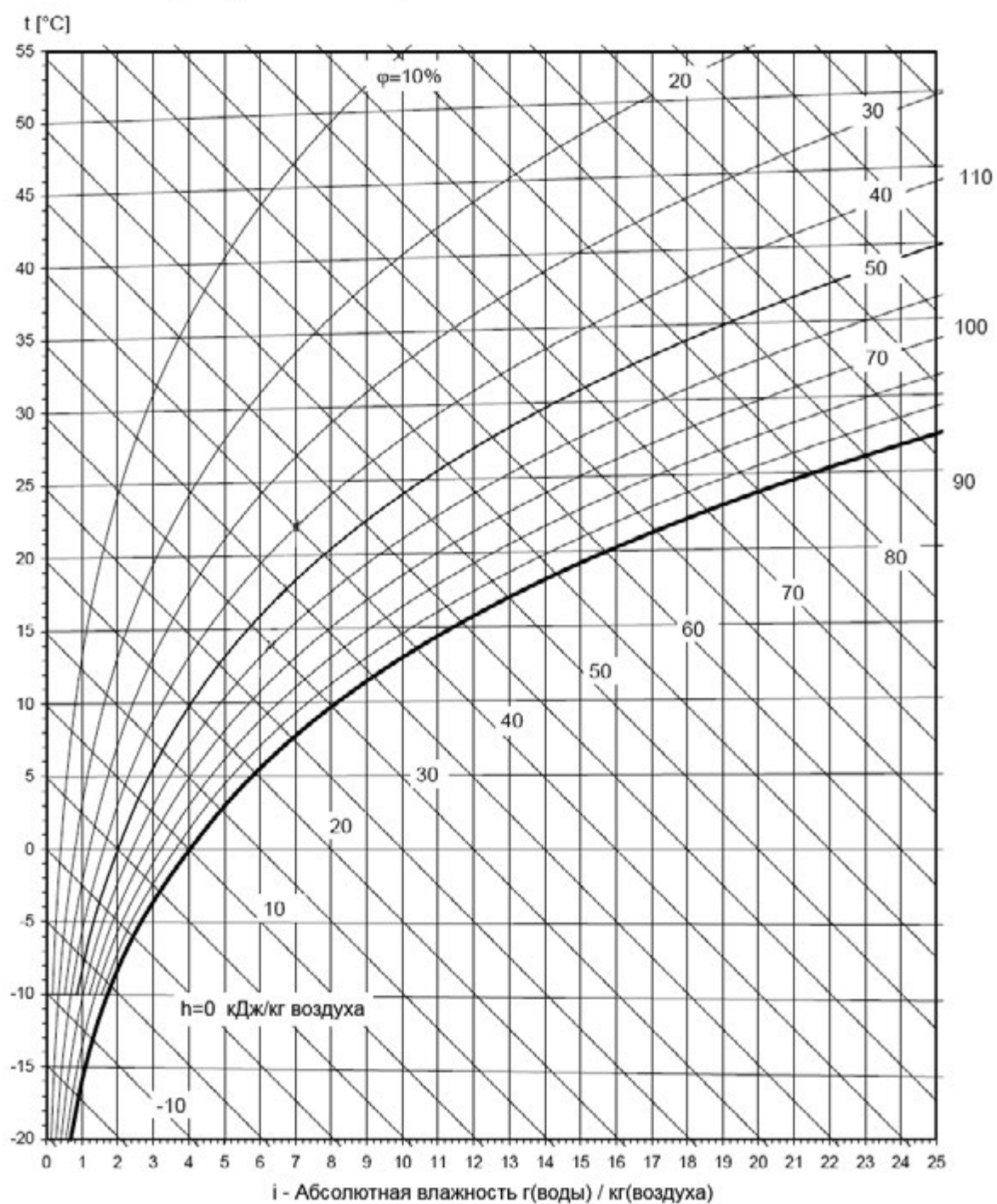
Тепловлажностная диаграмма (диаграмма Моляе)
