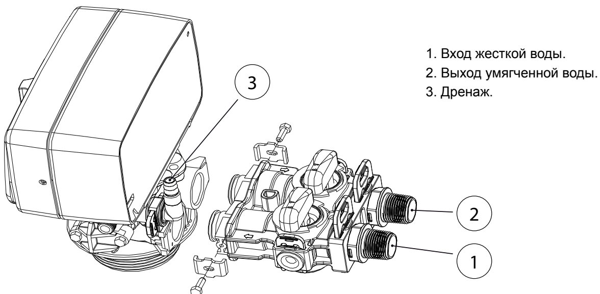
Рисунок 13 Гидравлические вход и выходы блока умягчения.
