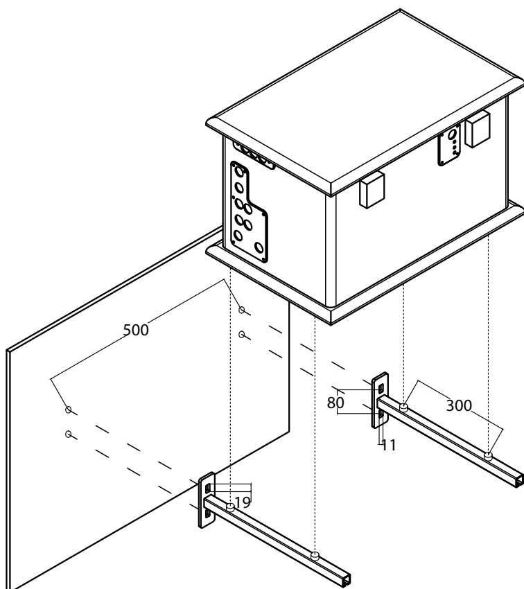
Рисунок 11 Схема монтажа центрального модуля системы увлажнения Buhler-AHS PG12UV.
