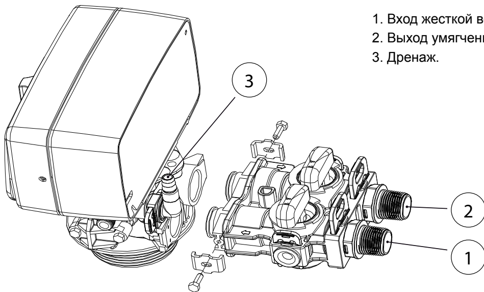
Рисунок 13 Гидравлические вход и выходы блока умягчения.
