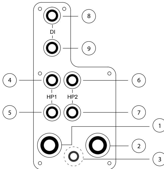
Рисунок 14 Панель гидравлических входов/выходов центрального блока увлажнения.
