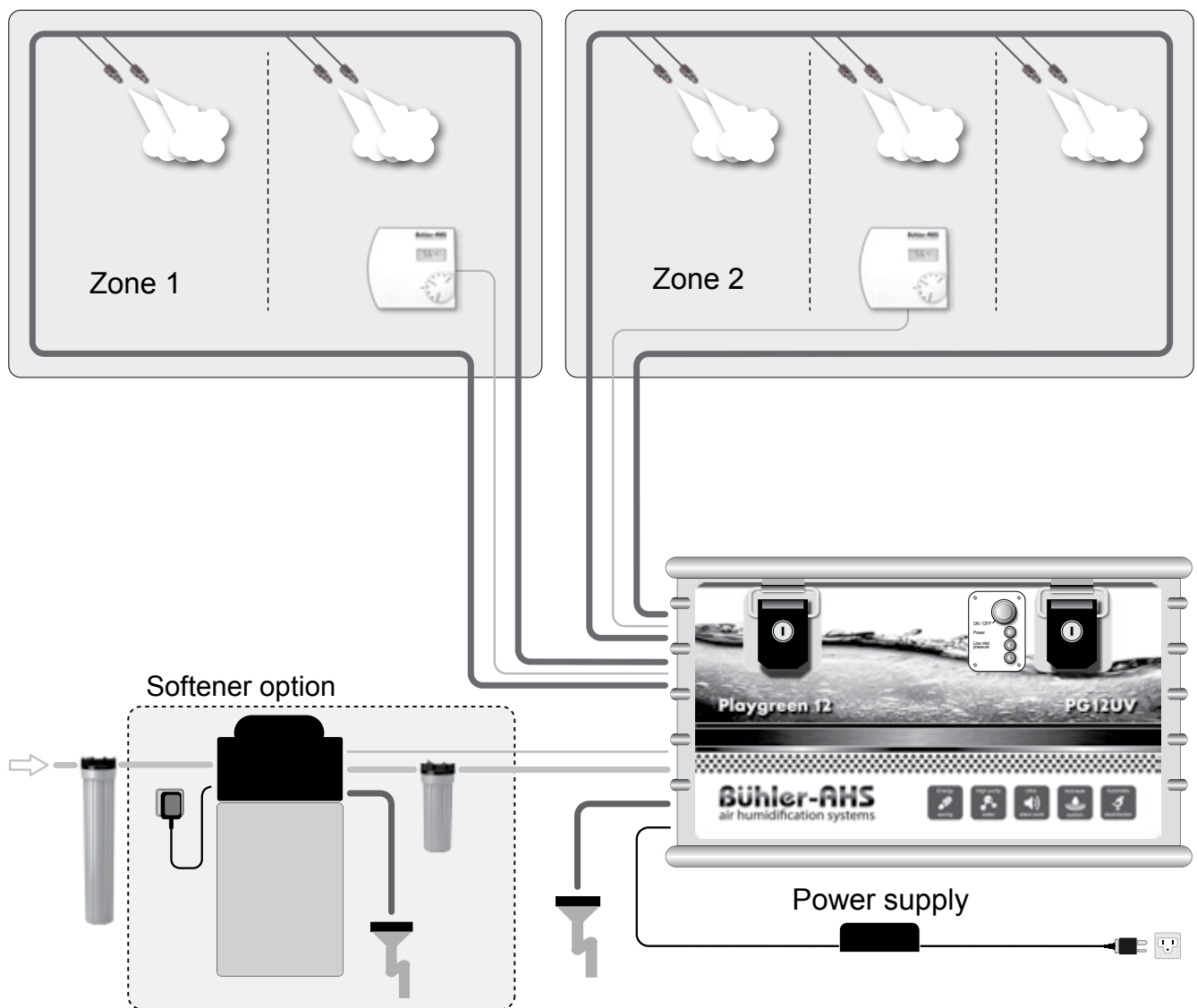
Рисунок 1 Структурная схема адиабатической системы увлажнения Buhler-AHS Playgreen 12.
