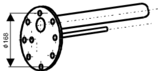
Фланец 2,2 кВт
