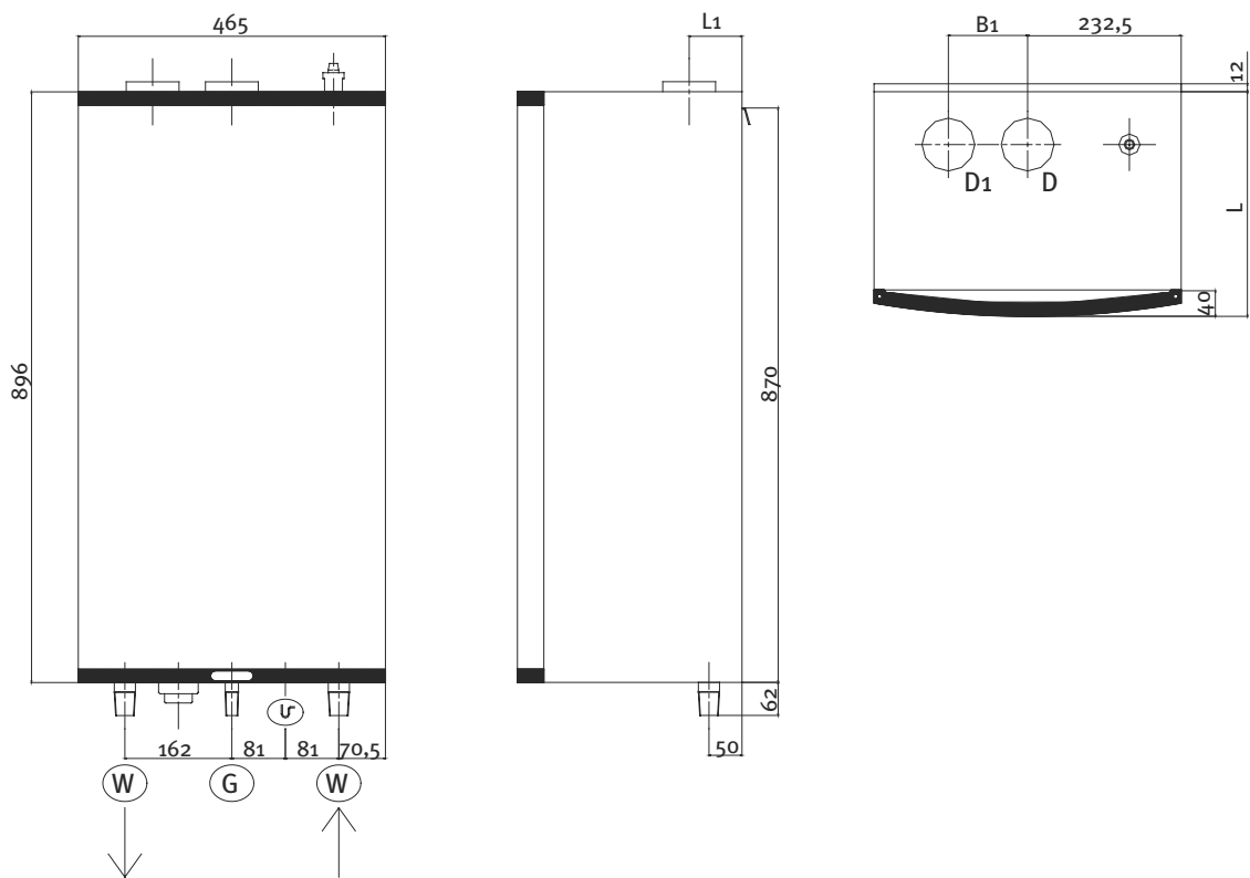
Рис. 1 Размеры R30
