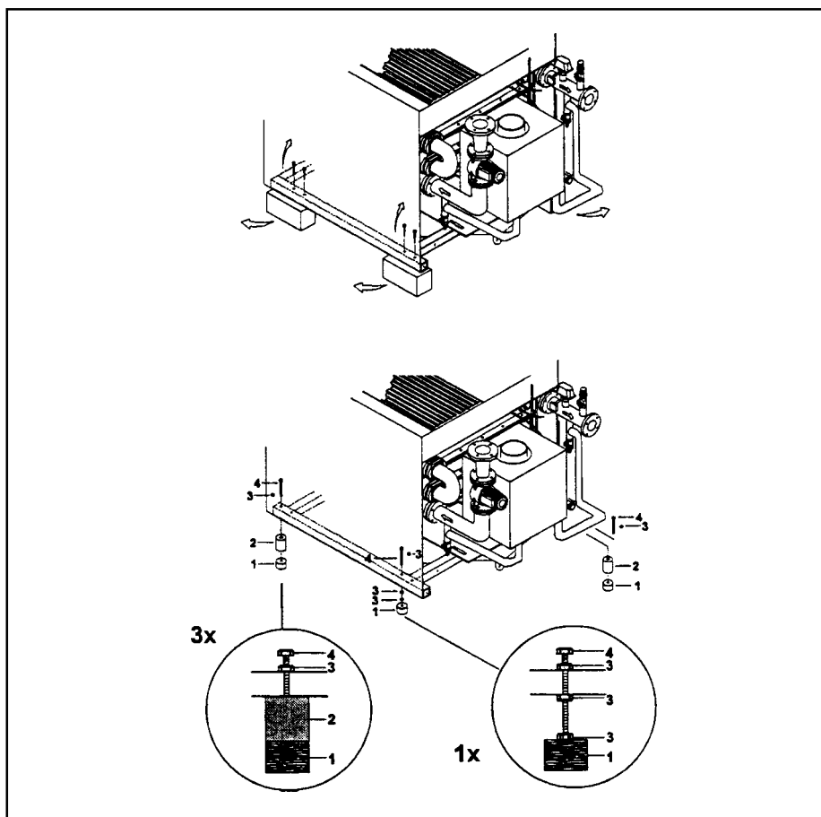
Рис. 13. Монтаж амортизаторов
