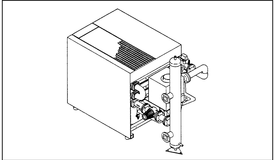
Рис. 28. Котел с установленным вертикально водосборником низкой скорости с правосторонними подключениями
