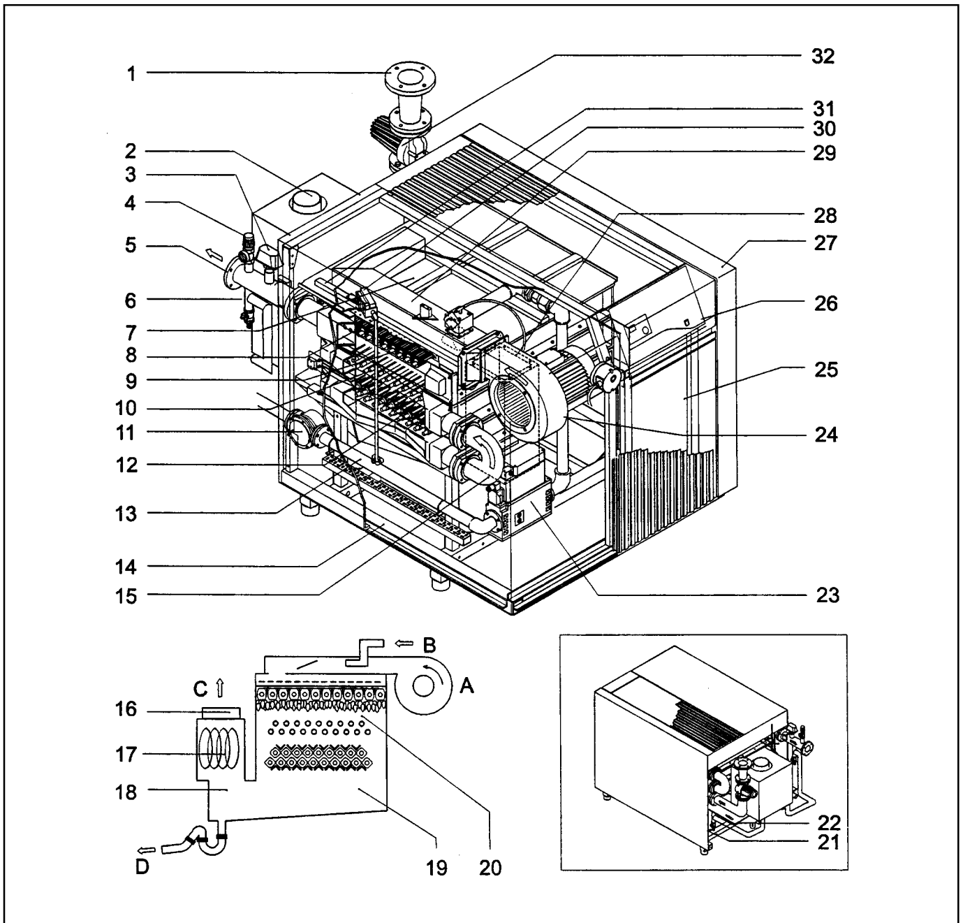
Рис. 5. Общий вид
