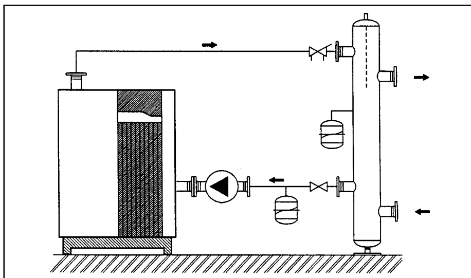
Рис. 27. Установка с водосборником низкой скорости, запорным клапаном и расширительным баком
