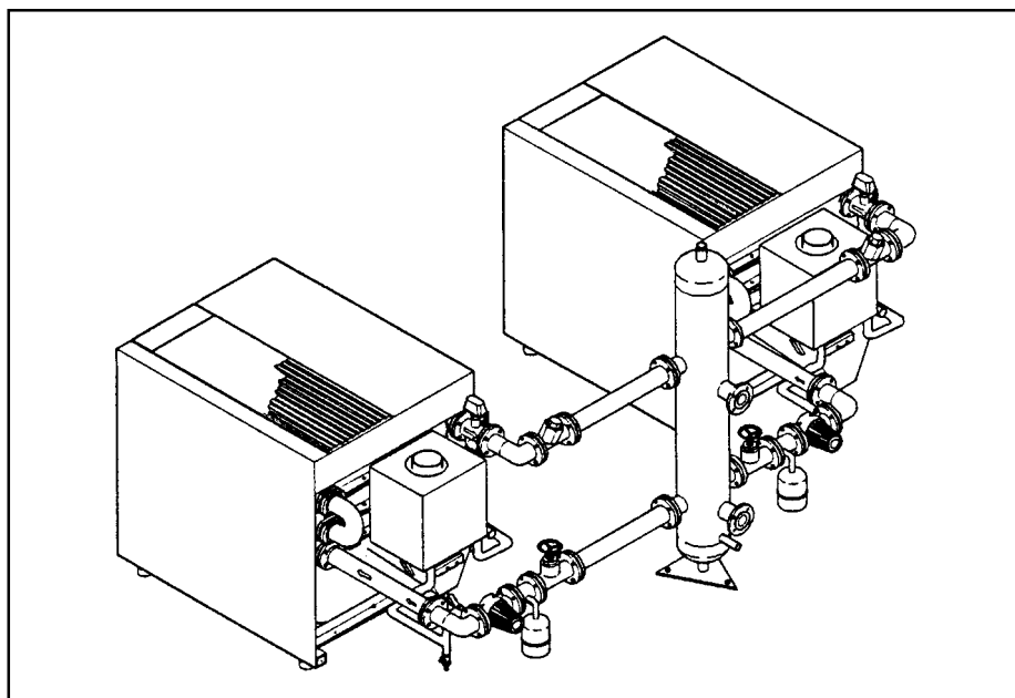
Рис. 31. Водосборник низкой скорости для двух котлов
