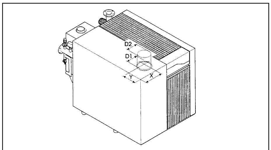
Рис. 19. Присоединение воздуховода
