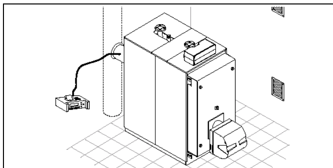
Охлаждение глазка пламени
