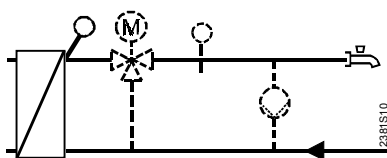
Установка без реле расхода
