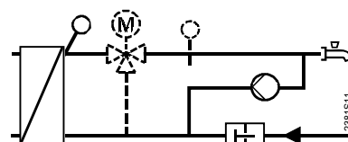
Установка с реле расхода
