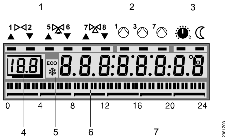
Дисплей контроллера RVD130(5)
