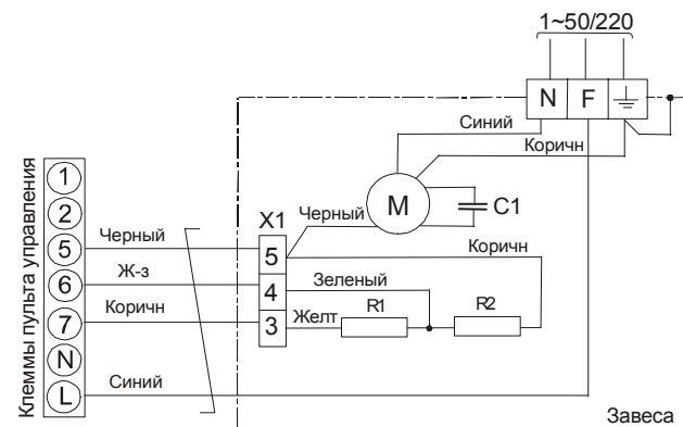
Рис. 2. Водяной воздушнонагреватель
