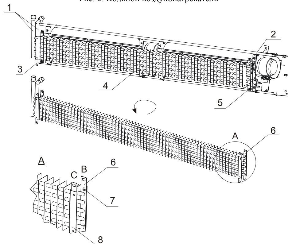
Рис. 2. Водяной воздушнонагреватель
