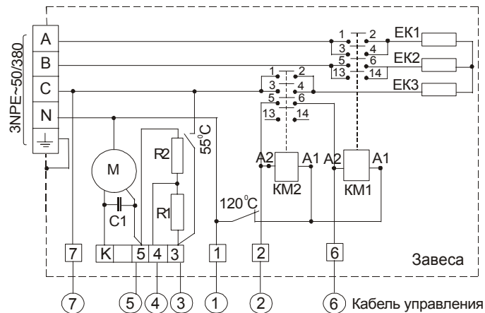
Рис. 1. Электрическая схема блока занавески
