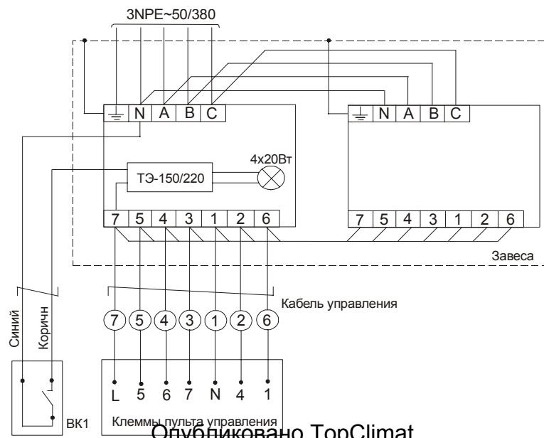
Рис. 2. Электрическая схема КЭВ-П601Е, КЭВ-П604Е*
