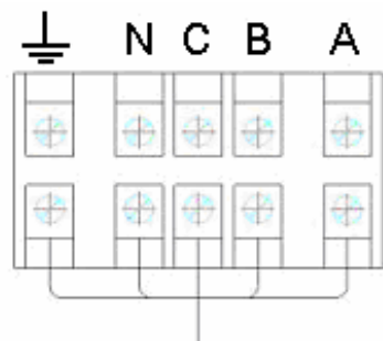
Рис. 9. Вид на клеммную колодку внутри корпуса завесы
