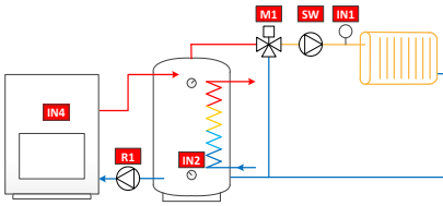
6. 1-контурная с системой горячей воды для бытовых нужд с норм. закрытым клапаном
