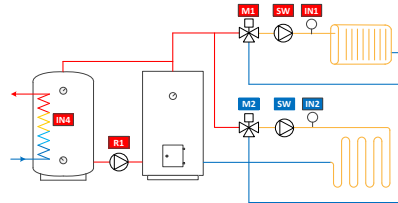
8. 2-контурная с системой горячей воды для бытовых нужд с норм. закрытым клапаном
