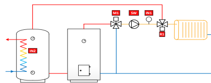
8. 2-контурная с системой горячей воды для бытовых нужд с норм. закрытым клапаном
