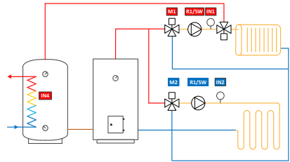
10. 1-контурная с ограничением температуры возвратной воды
