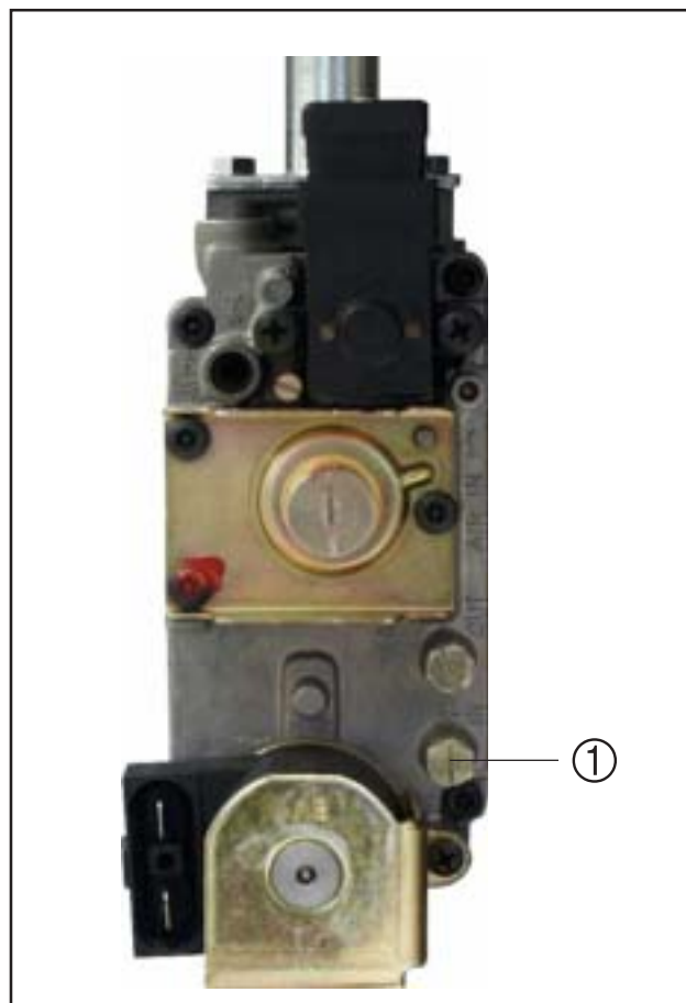
Рис.: Удалить воздух, проверить давление подключения газа
