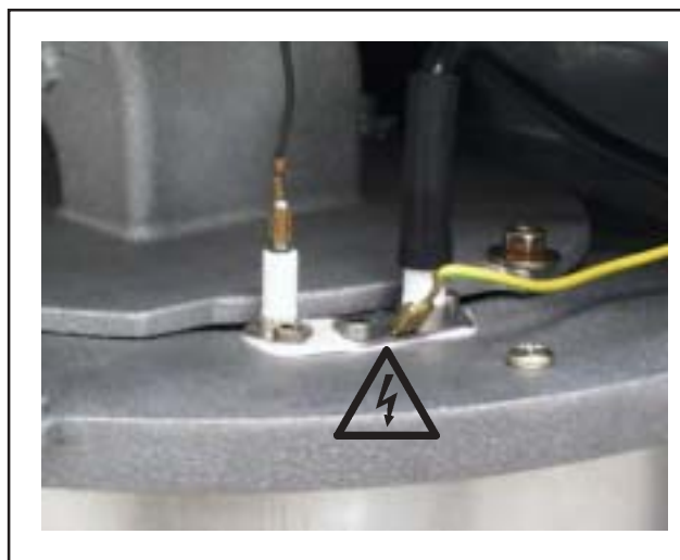
Рис.: Электрод поджига Опасность от электрического напряжения
