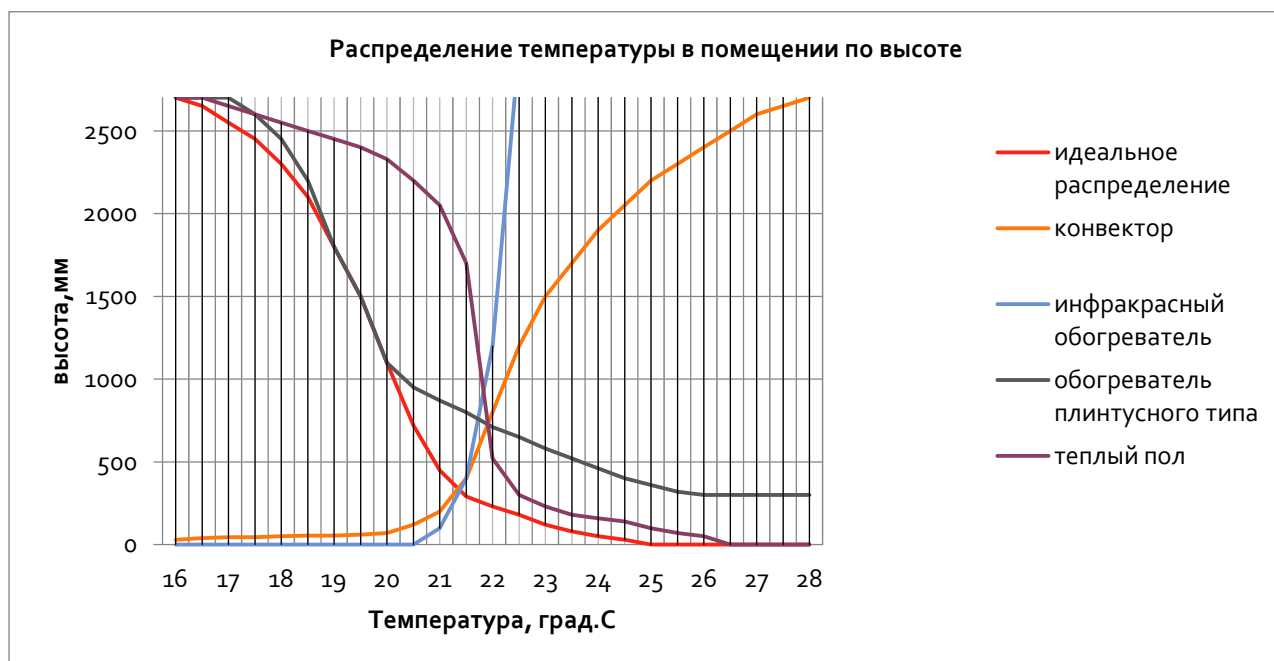
Рис. 11. Распределение температуры в помещении по высоте.
