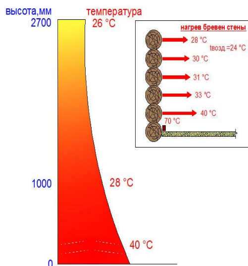
Рис. 9. Принцип работы плинтусного обогревателя.
