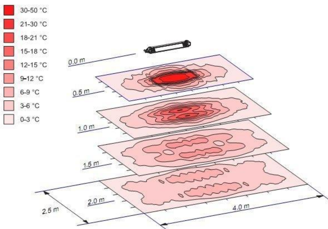
Рис. 3. Распределение температур инфракрасного обогревателя в зависимости от расстояния по вертикальной оси и высоты установки обогревателя
