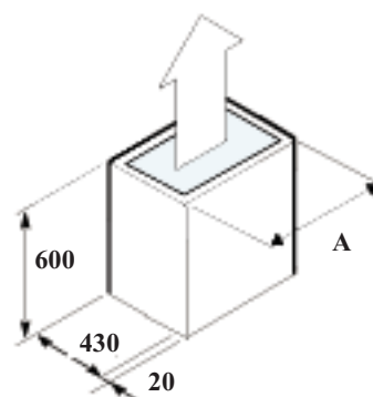
Звукоизолированная воздушораспределительная камера
